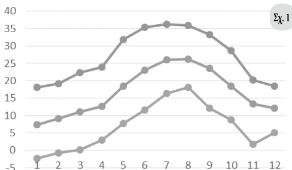
Σχ. 1. Η ετήσια πορεία της θερμοκρασίας του αέρα (°C) στην Κασσάνδρεια (μέγιστες, μέσες και ελάχιστες τιμές) κατά το έτος 2020.
