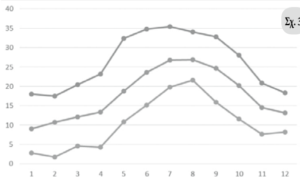
Σχ.3 Η ετήσια πορεία της θερμοκρασίας του αέρα στον Ν. Μαρμαρά (μέγιστες, μέσες και ελάχιστες τιμές) κατά το έτος 2020.
