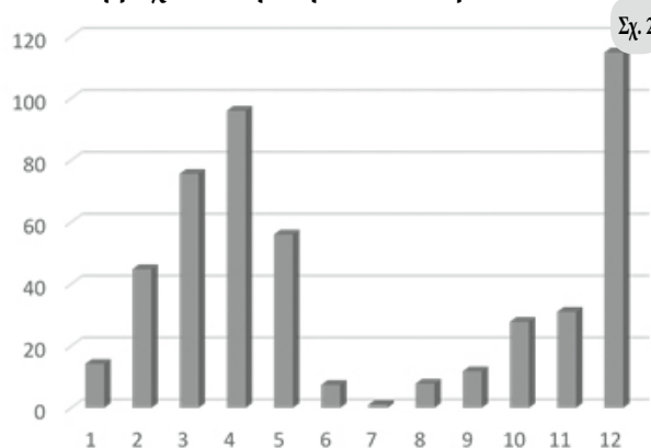
Σχ. 2. Η ετήσια πορεία της βροχής (mm) στην Κασσάνδρεια κατά το έτος 2020
